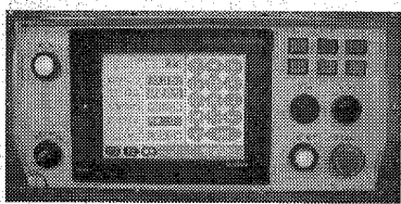
＜テンキー式角度設定方式＞
